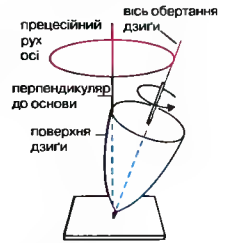
Пресесія Вісь обертання дзиги окреслює конічну поверхню
